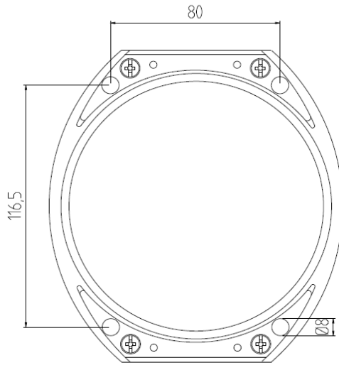
Bild 77: Maße der Montagelöcher
