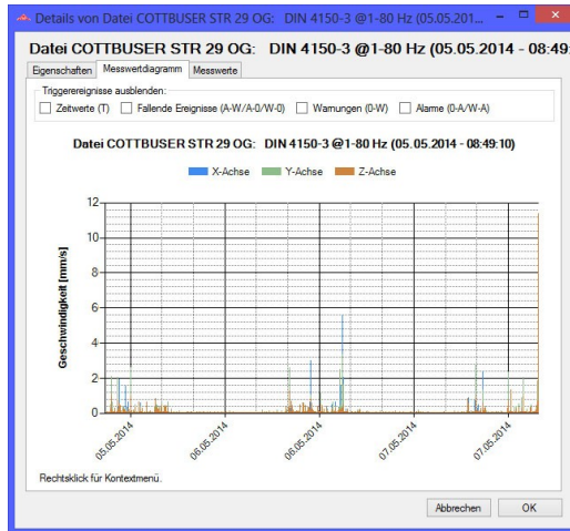
Bild 69: Messwertdiagramm
